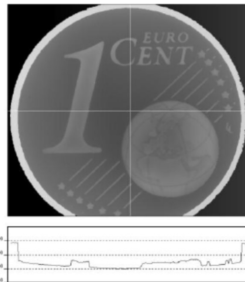
Změřený výškový profil mince (výšková mapa)
